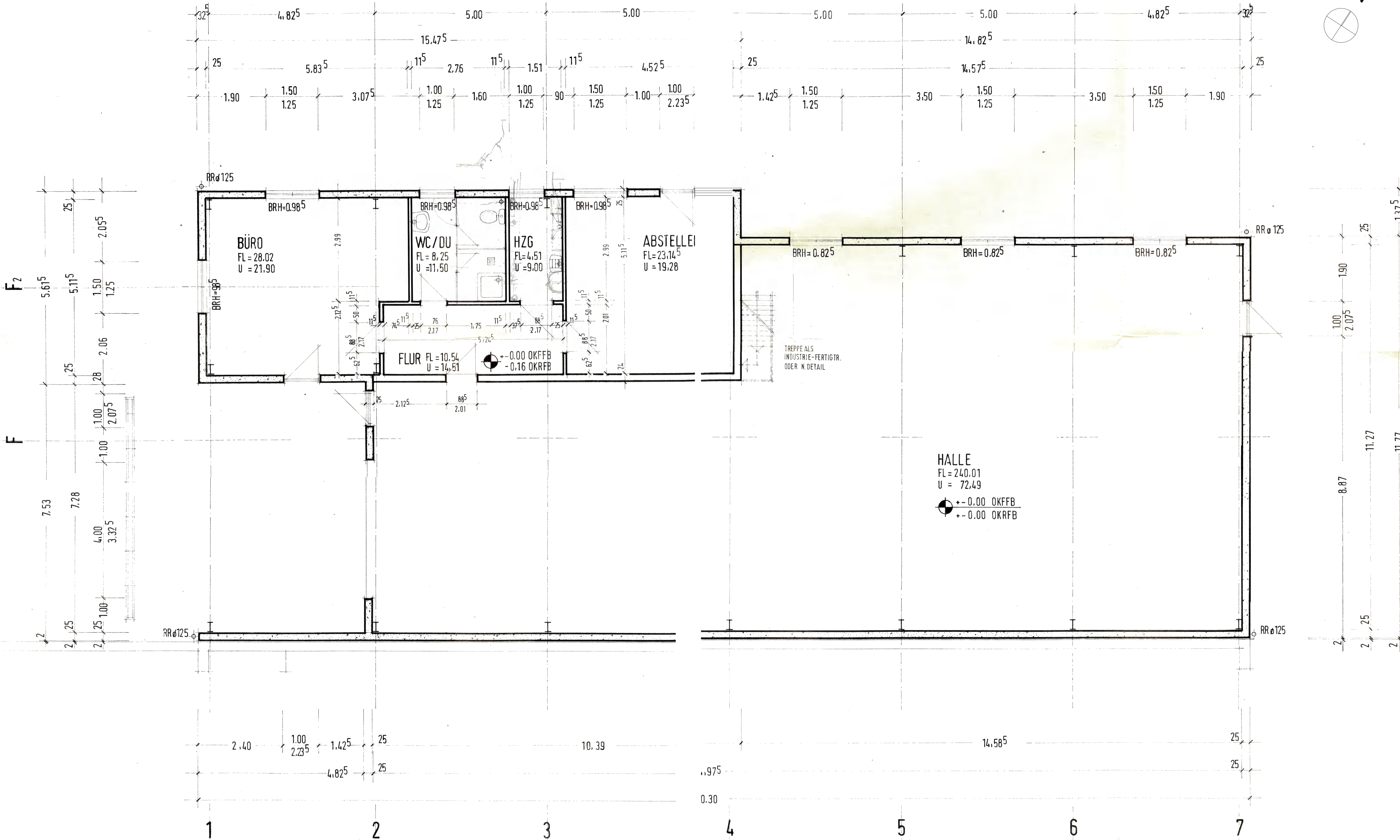
Grundriss - Entwässerungsplanung
