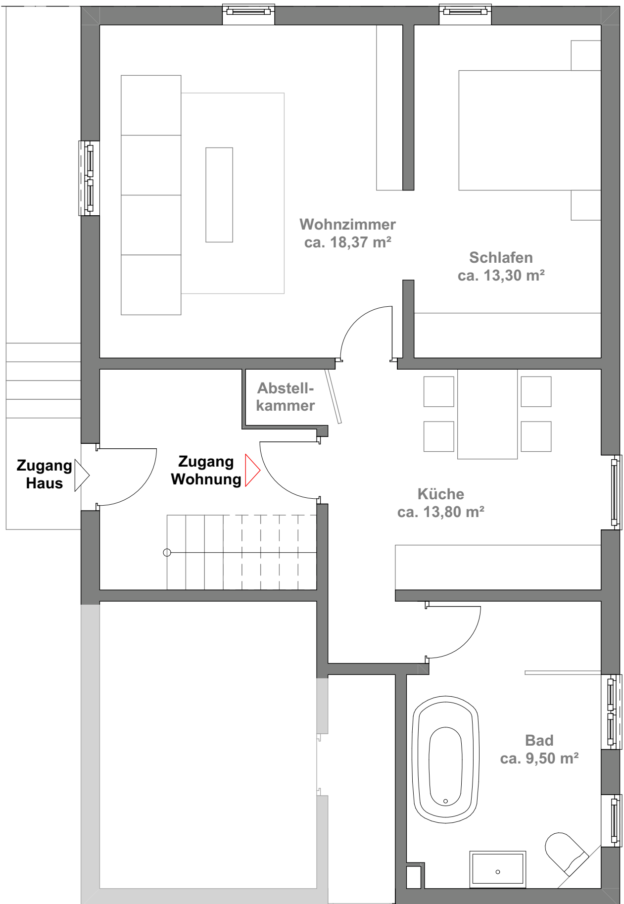
Grundriss Erdgeschoss
