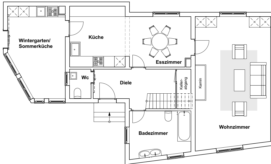
Grundriss Erdgeschoss
