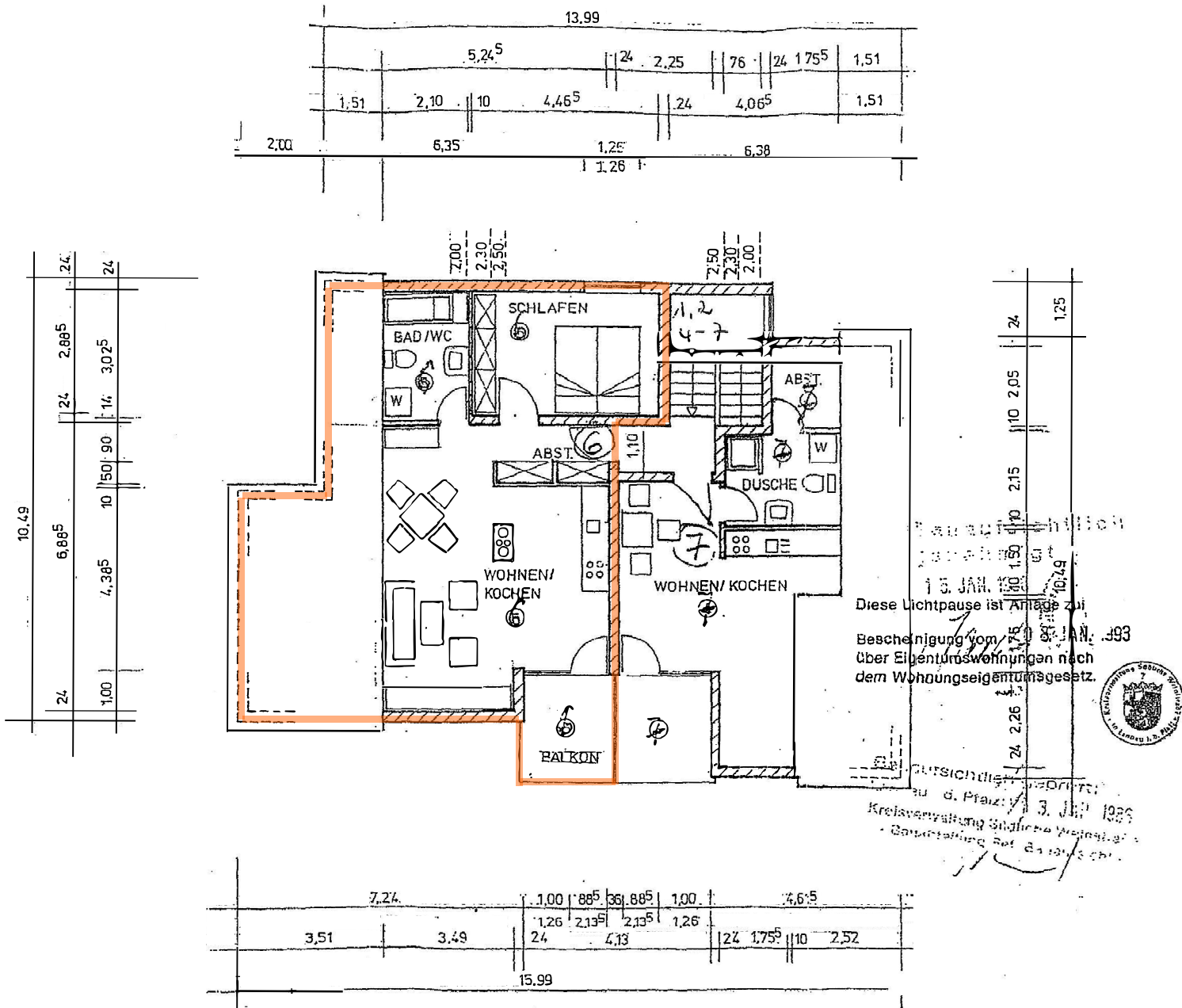
Dachgeschoss
